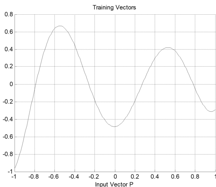
Рисунок 5.8 – Графік функції апроксимації при значенні SPREAD=1
